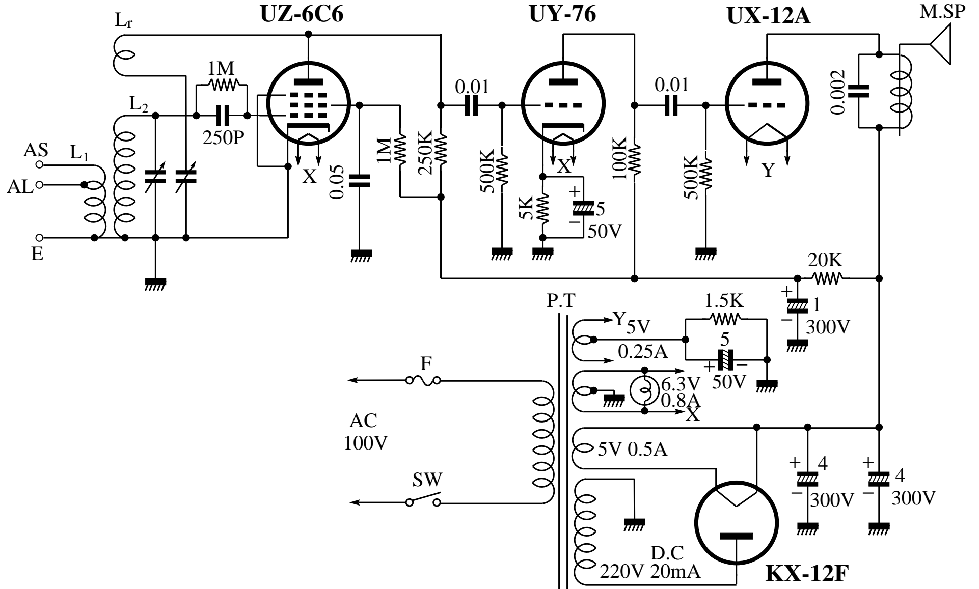
並 4 球受信機 (6C6-76-12A-12F) 『ラジオ技術教科書』 所収
