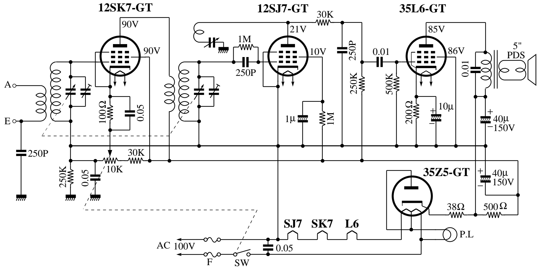
GT 管使用高トランスレス 4 球受信機 (12SK7-12SJ7-35L6-35Z5) 『ラジオ技術教科書』 所収
